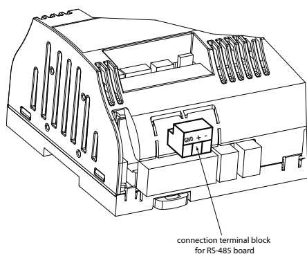
Рис. 5.d (детализация электронной платы, электрическая секция увлажнителя)
